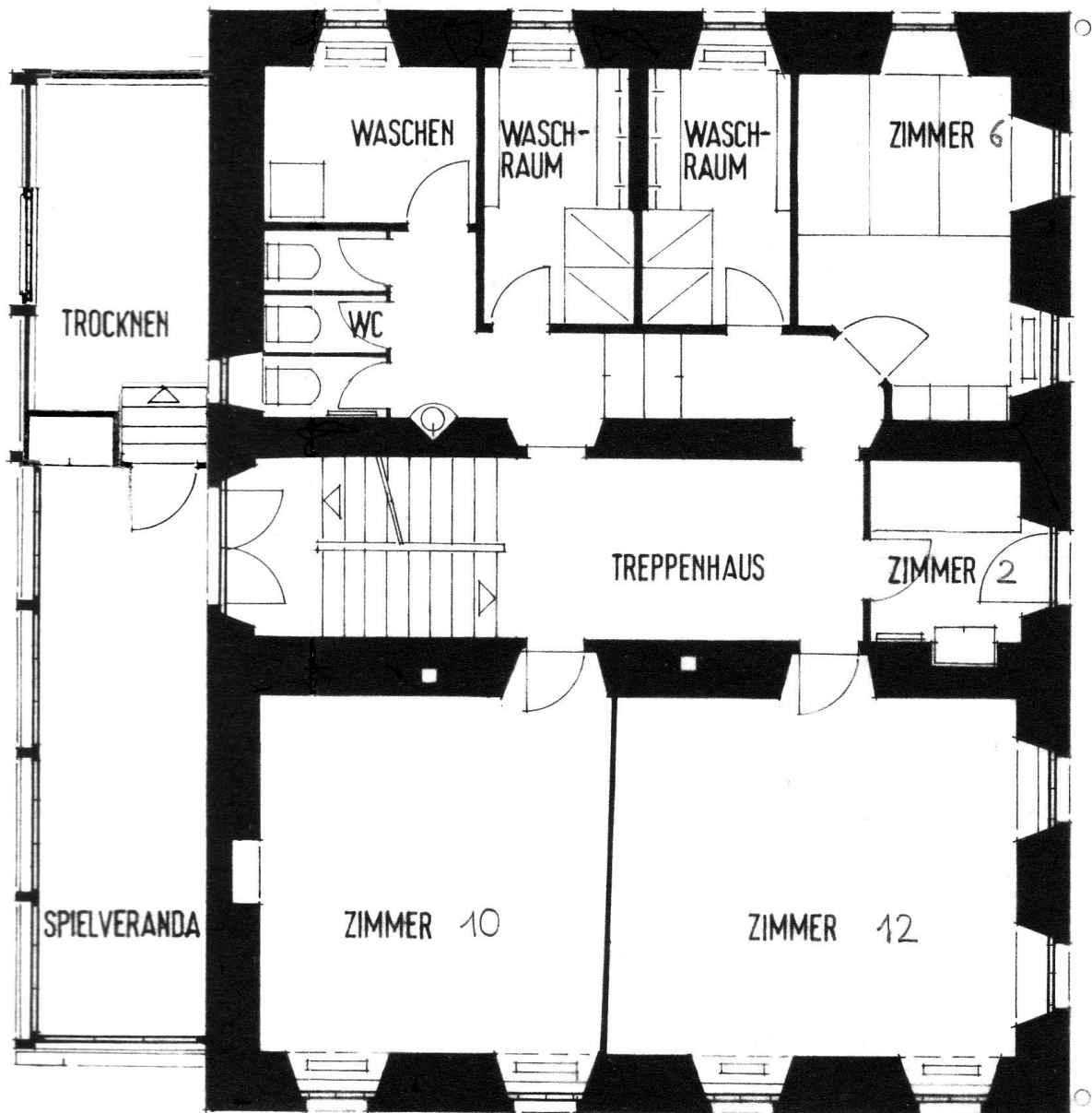
1. OBERGESCHOSS
