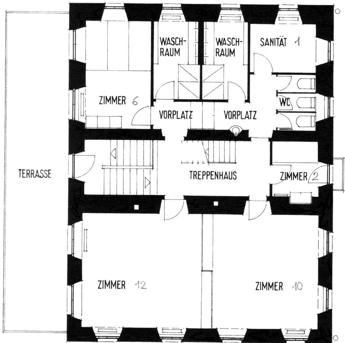
2. OBERGESCHOSS
